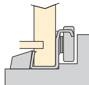
Esquema de montaje de la guía al cajón. Esquema de montagem da corrediça à gaveta.
